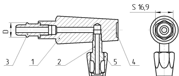
Рис.1 Штекер газовый ДЖЕТ 294 01 00 00;-01
