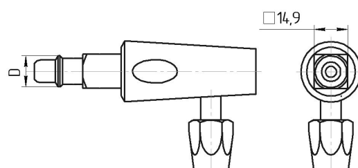
Рис.3 Штекер газовый ДЖЕТ 294 01 00 00-03;-04
