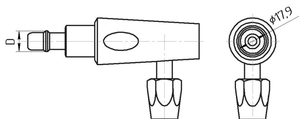
Рис.1 Штекер газовый ДЖЕТ 294 01 00 00;-01
